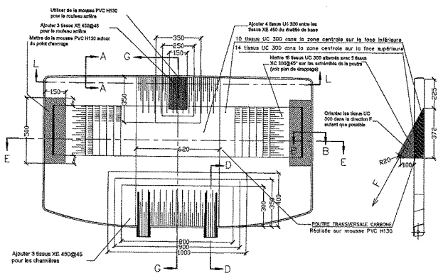
STRUCTURE PORTE COMPOSITE Échelle: 1/10
